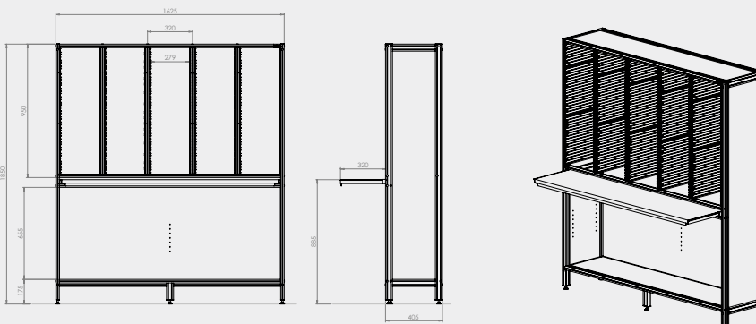
Verdeelstation 5 koloms
