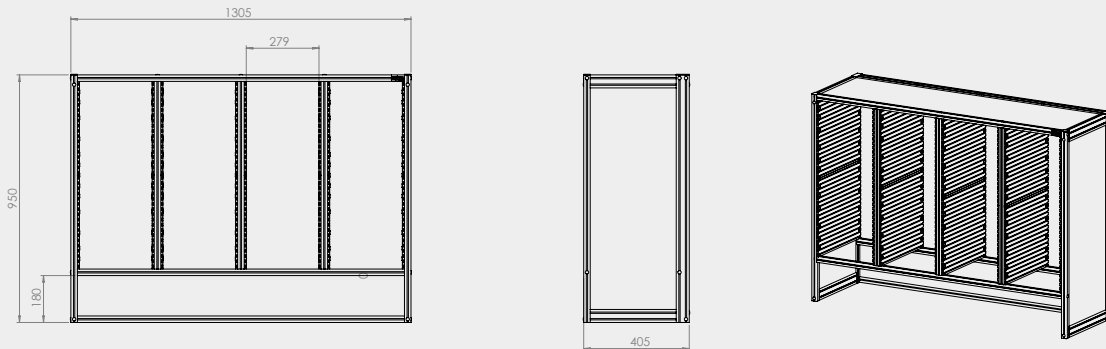
Sorteerunit 4 koloms
