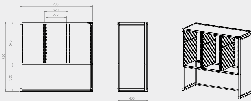
Sorteerunit 3 koloms
