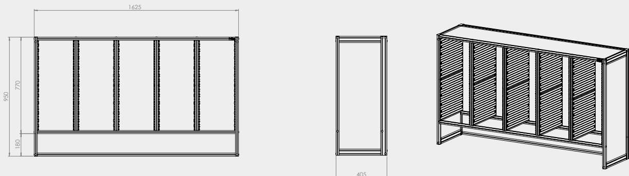
Sorteerunit 5 koloms
